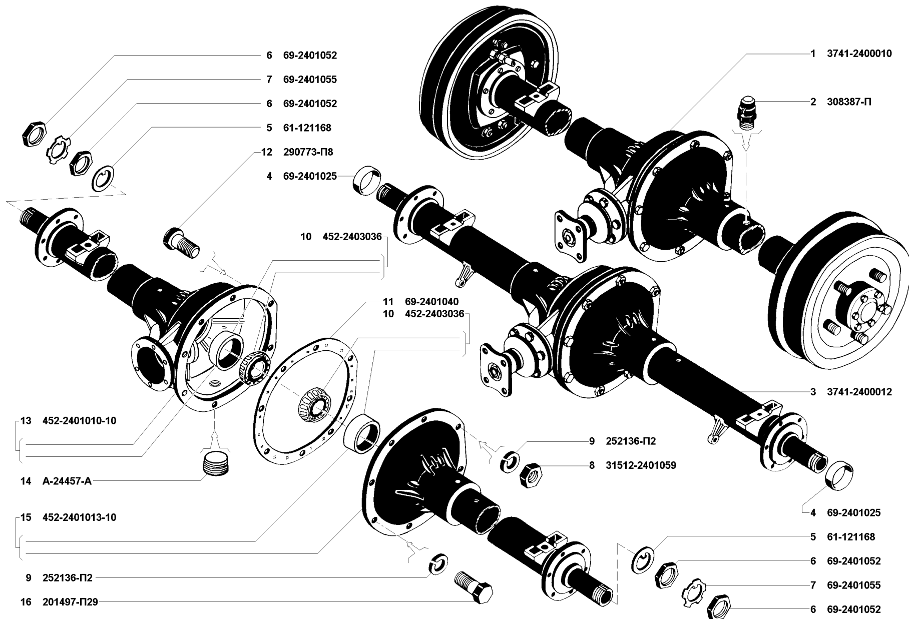
Рис. 63. Мост задний ведущий в сборе (2400), картер и кожухи полуосей заднего моста (2401)
