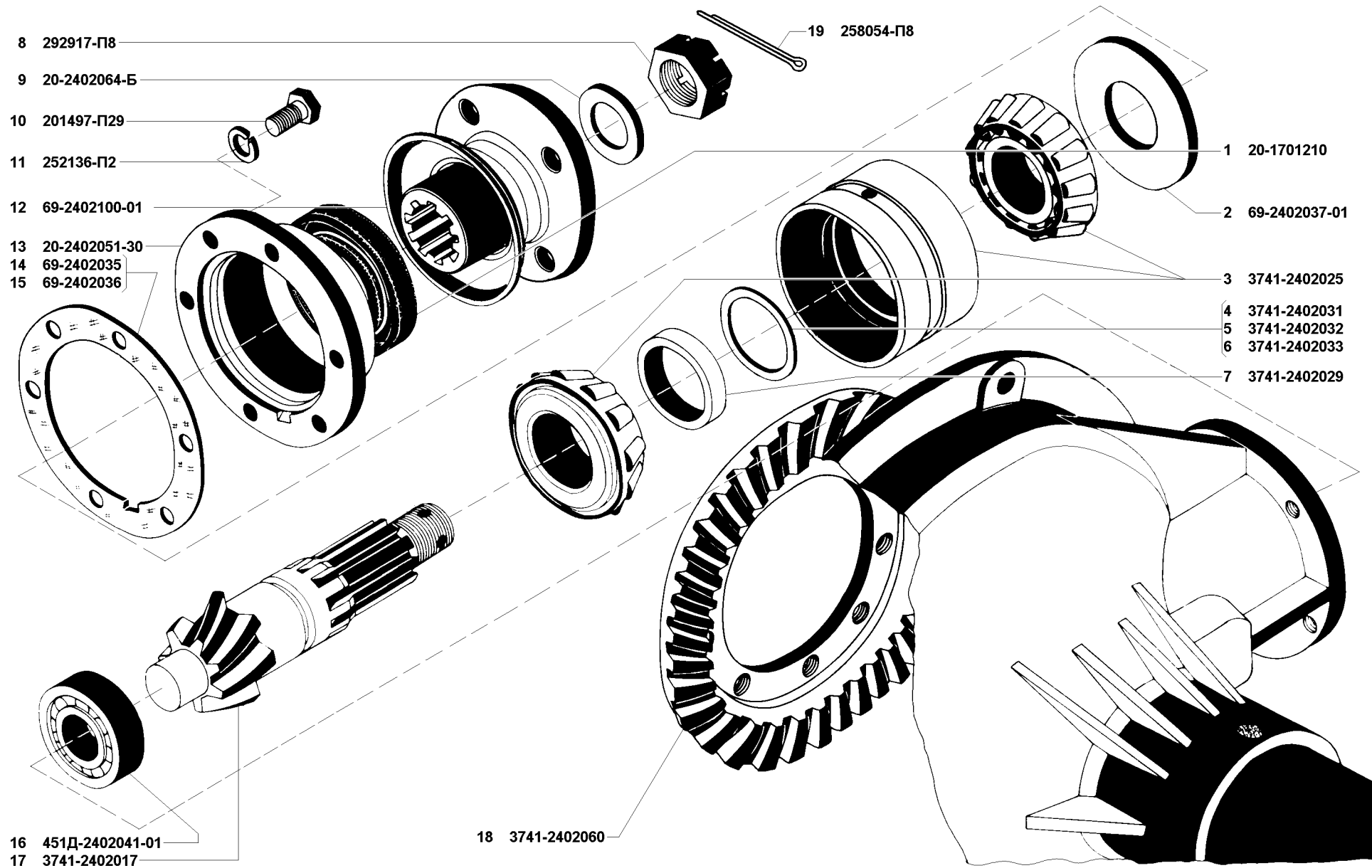
Рис. 64. Передача главная переднего и заднего мостов (2402)
